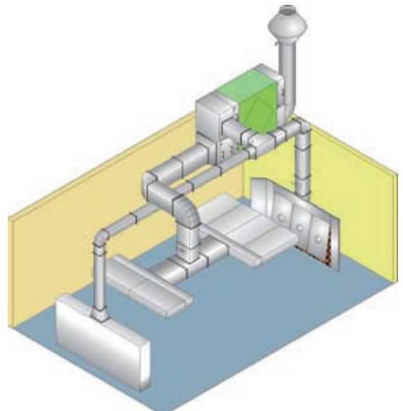
Beispiel mit einem zusätzlichen Trockenbereich und einer Wärmerückgewinnungsanlage.
